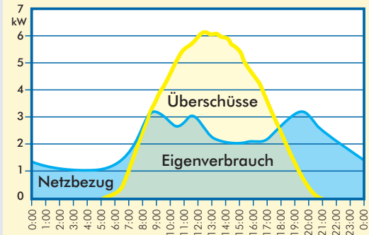
Typischer Stromlastgang eines landwirtschaftlichen Betriebs mit einem Jahresstrombedarf von 20.000 kWh, 7 kW Photovoltaik-Anlage
